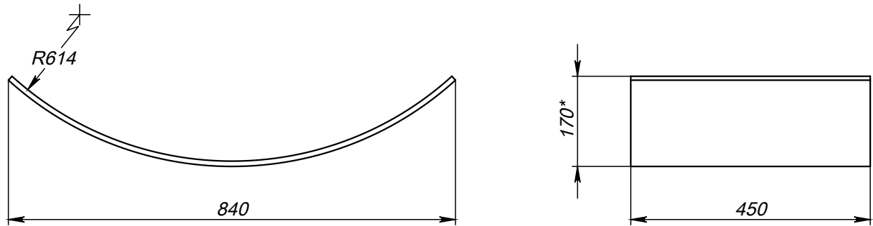
Поз.3 (Ложемент)
